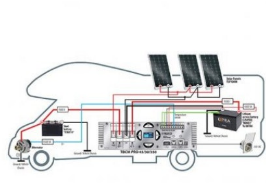
Utilisation du chargeur Teleco TBCM PRO 45/30/350© DR
